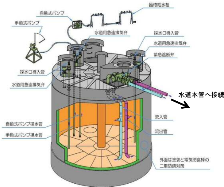
飲料水兼用耐震性貯水槽(イメージ)
