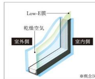
Low-E複層ガラス
