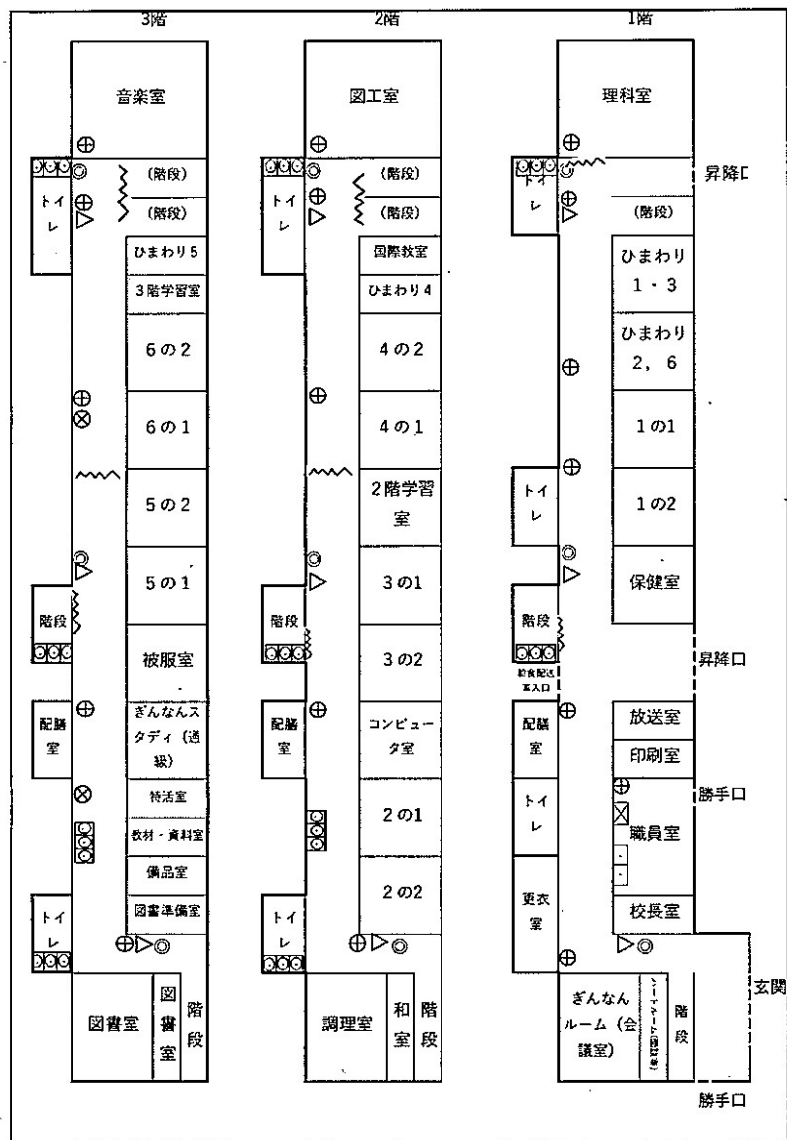
校舎内教室等配置図
