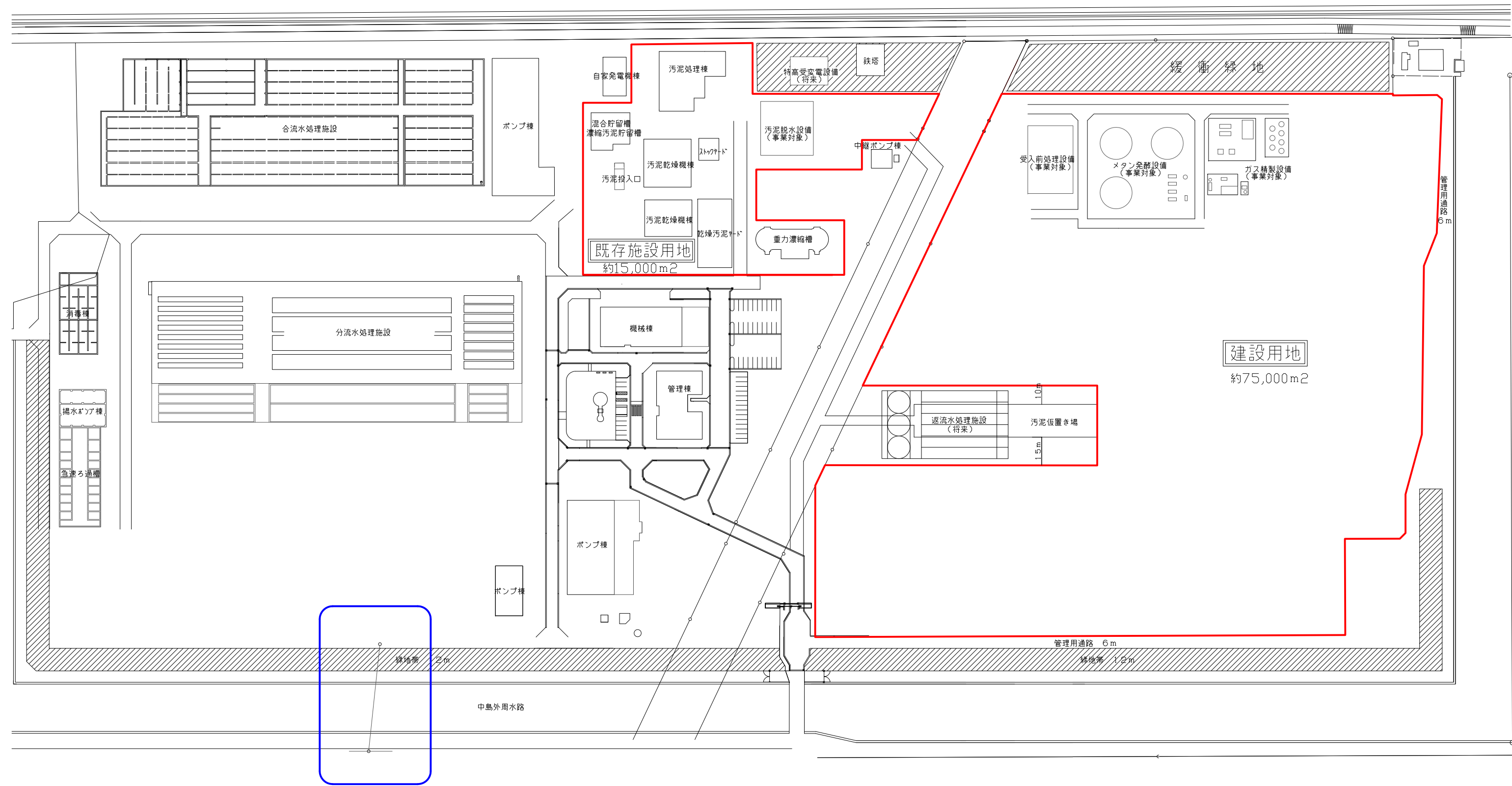
中島処理場受電引き込み位置 (6 kV)
