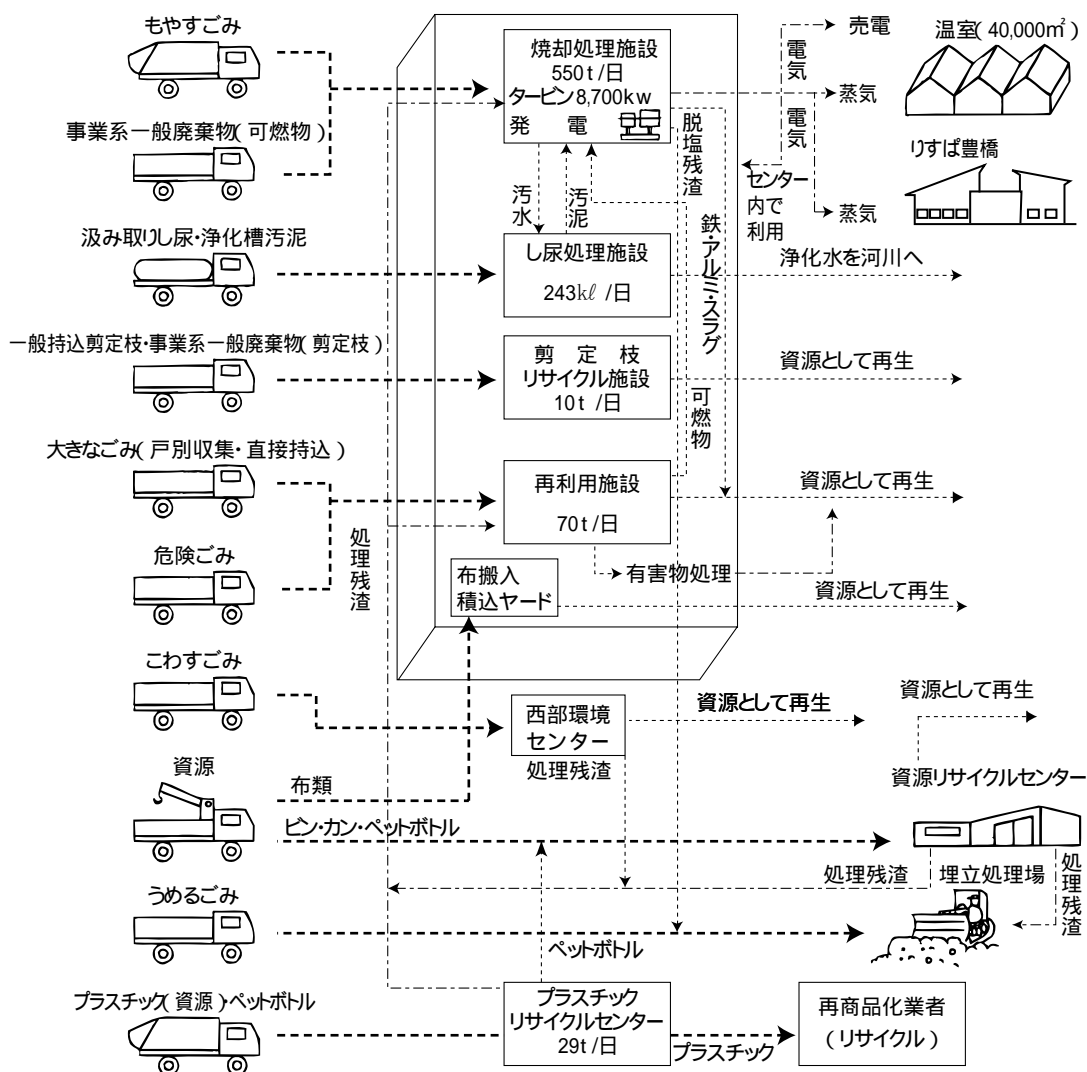
中間処理施設等概念図
