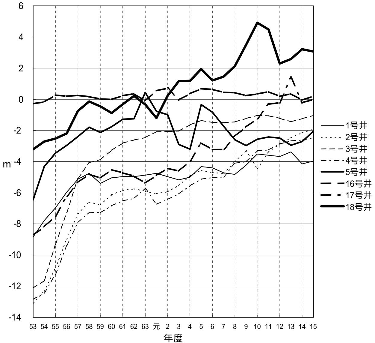
図2 - 生 - 23 地下水位 (東京湾中等潮位からの水位、一部井戸省略)
