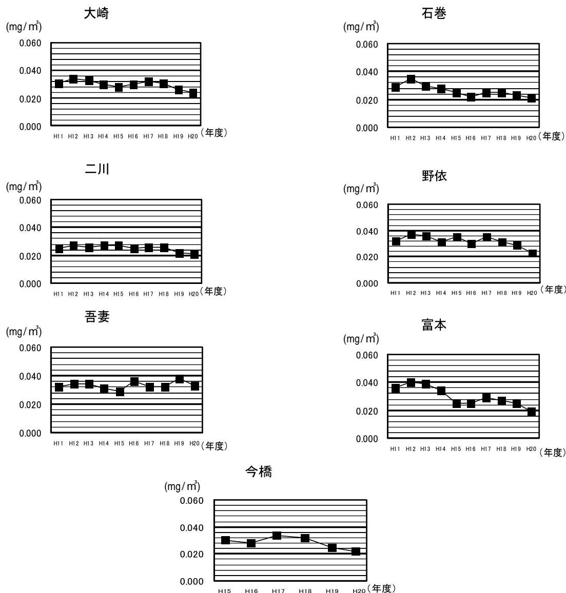
浮遊粒子状物質経年変化（平成11年度～平成20年度） （今橋は平成15年度～平成20年度）
