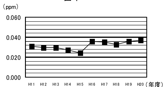
光化学オキシダント経年変化（平成 11 年度～平成 20 年度） 吾妻 富本
