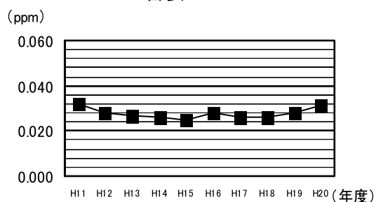
光化学オキシダント経年変化（平成 11 年度～平成 20 年度） 吾妻 富本
