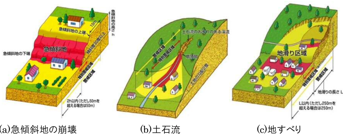
図-1.5 土砂災害警戒区域と土砂災害特別警戒区域(イメージ)
