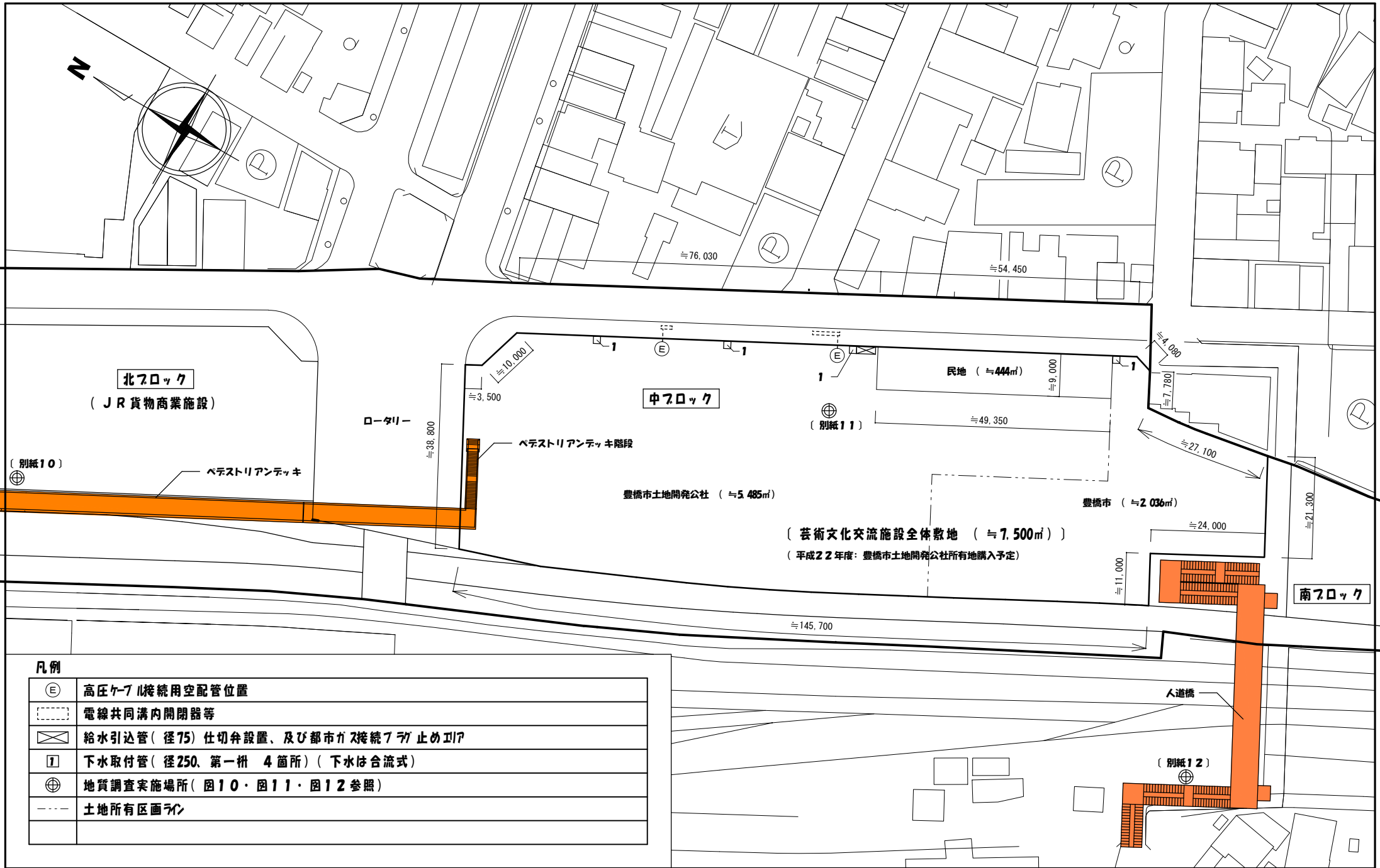
( 別紙2 ) 敷地詳細図 1/1,000
