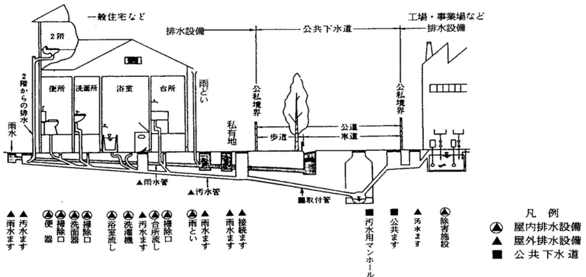
図 4-1-1 排水設備の例（分流式：公共下水道） （下水道排水設備指針と解説－2016年版－）
