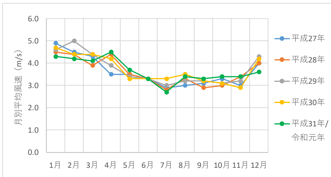
図 3-1-4 豊橋地域気象観測所における月別平均風速（平成 27～31 年/令和元年）の変化
