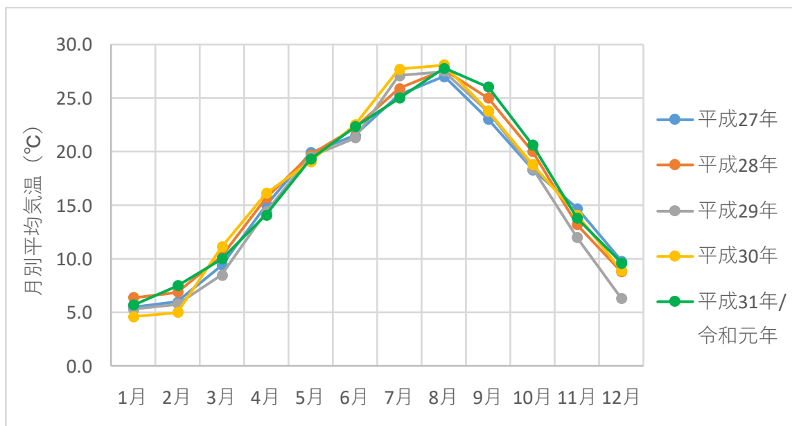
図3-1-2 豊橋地域気象観測所における月別平均気温（平成27～31年/令和元年）の変化
