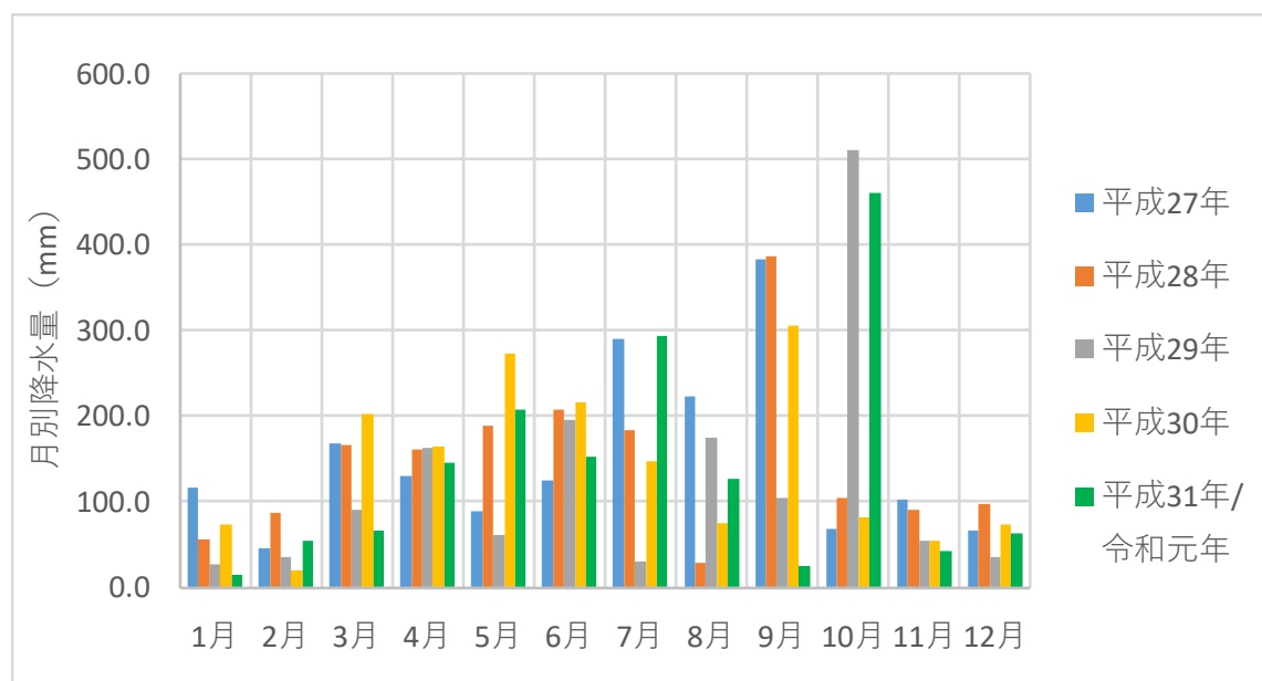
図3-1-3 豊橋地域気象観測所における月別降水量（平成27～31年/令和元年）の変化
