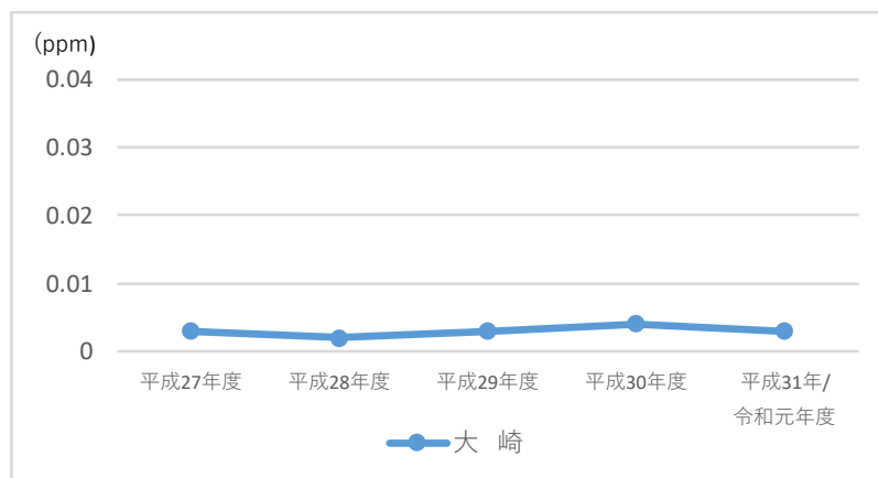
図 3-1-14 二酸化硫黄の経年変化（日平均値の2%除外値）
