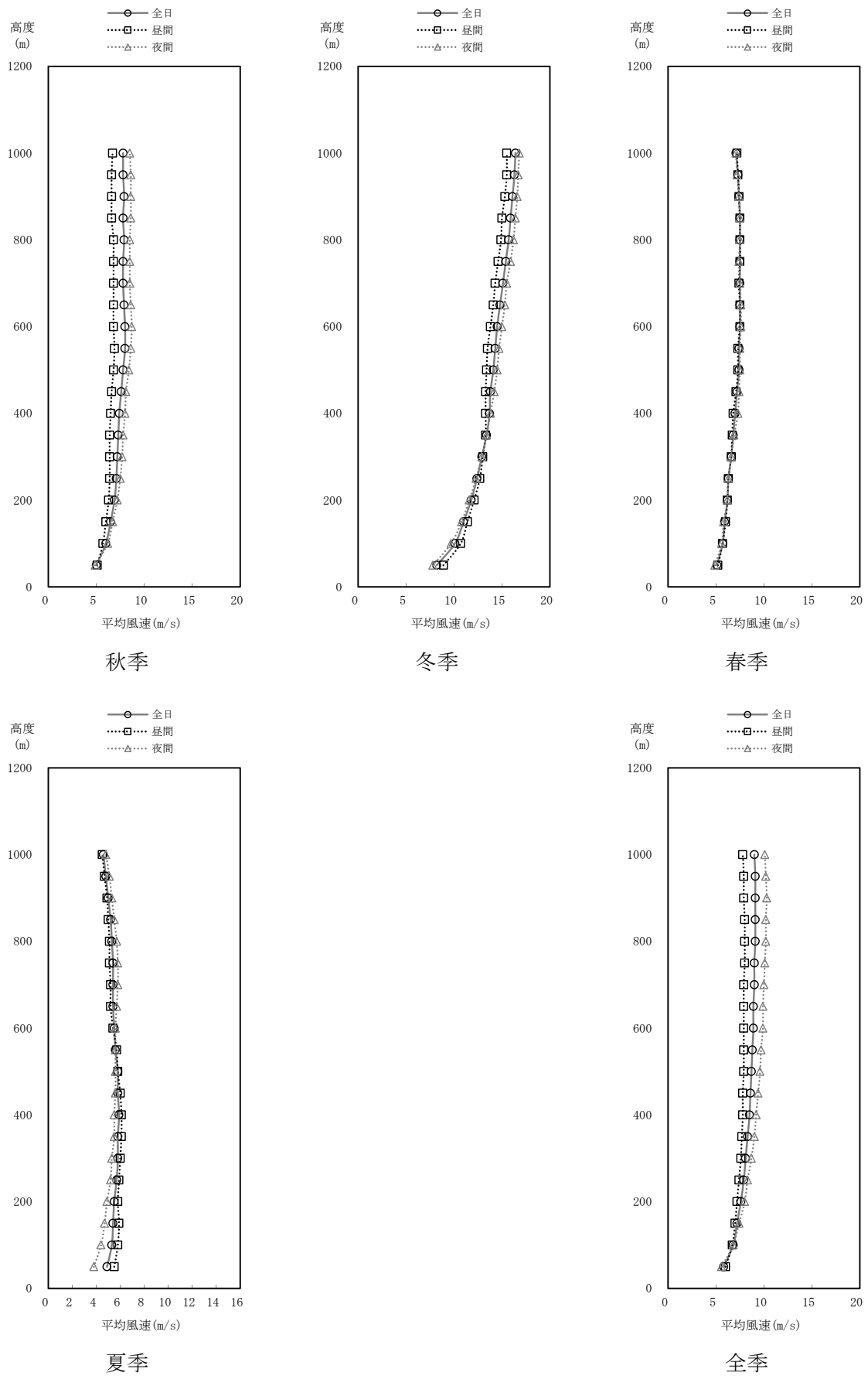
図3-1-10 高度別平均風速
