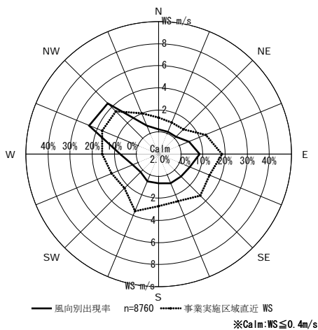
図3-1-8(2) 年間風配図 (通年調査)
