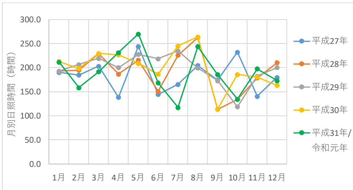
図3-1-6 豊橋地域気象観測所における月別日照時間（平成27～31年/令和元年）の変化
