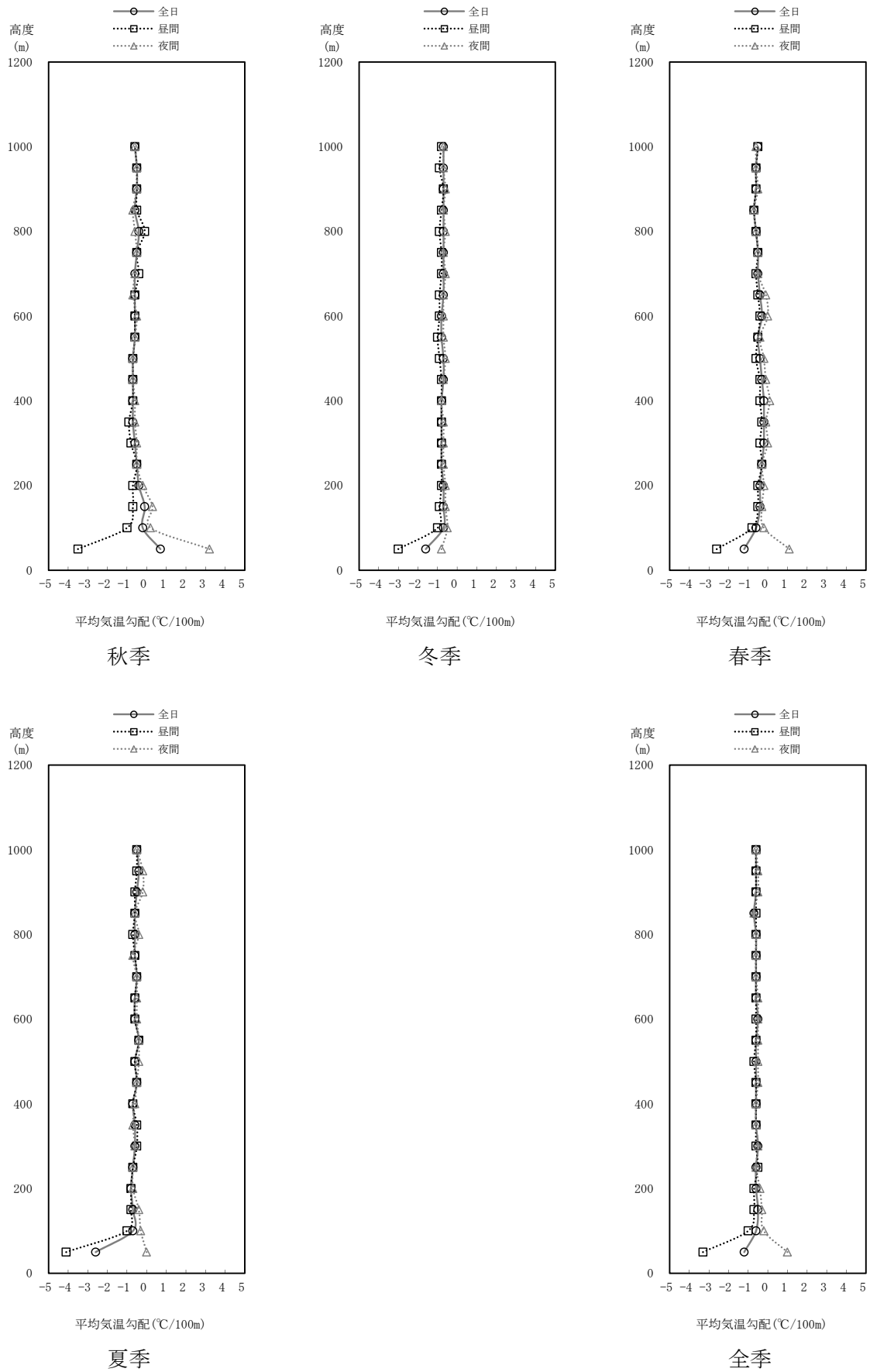
図3-1-12 高度別平均気温勾配
