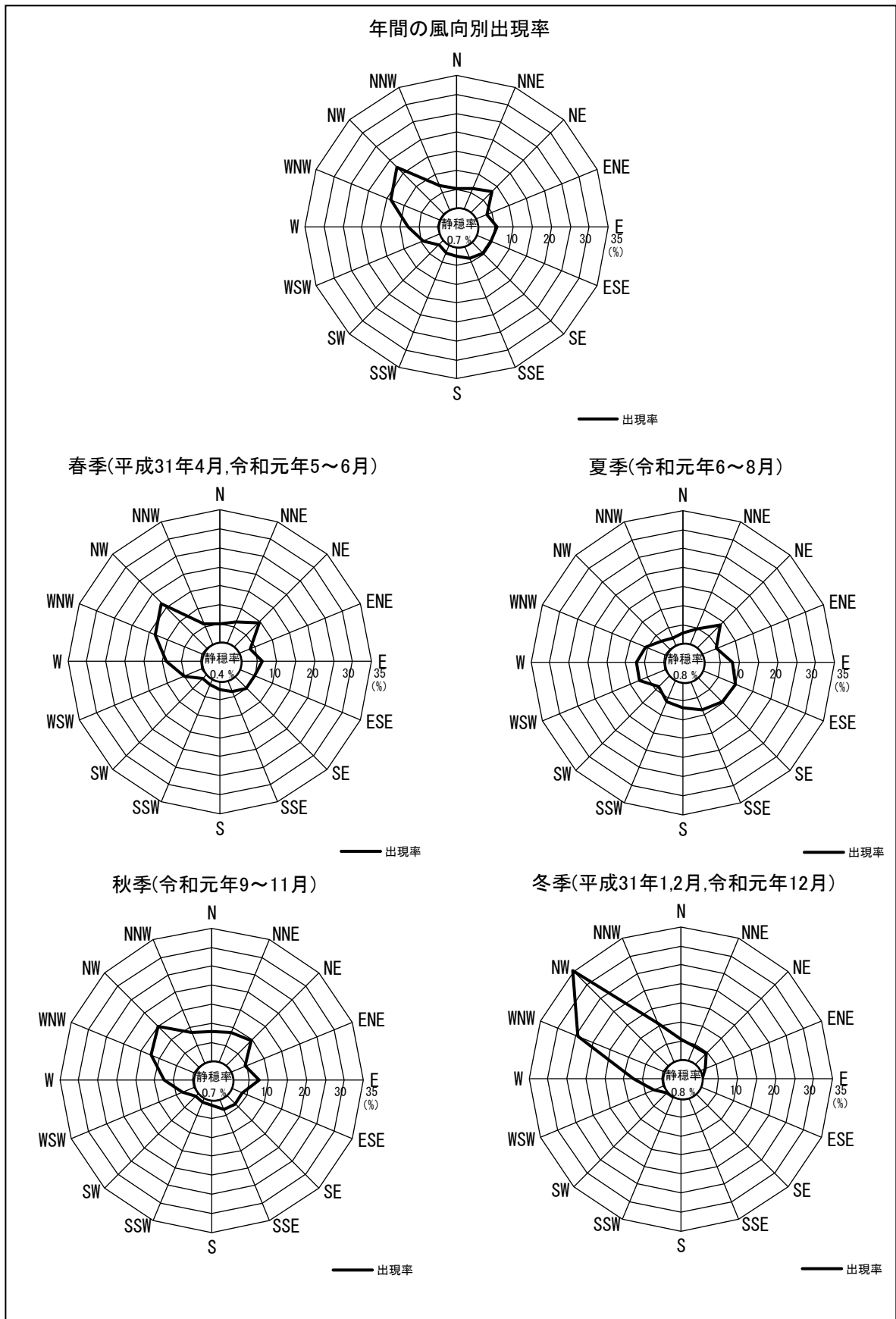
図 3-1-5 豊橋地域気象観測所における風配図 (平成 31 年/令和元年)
