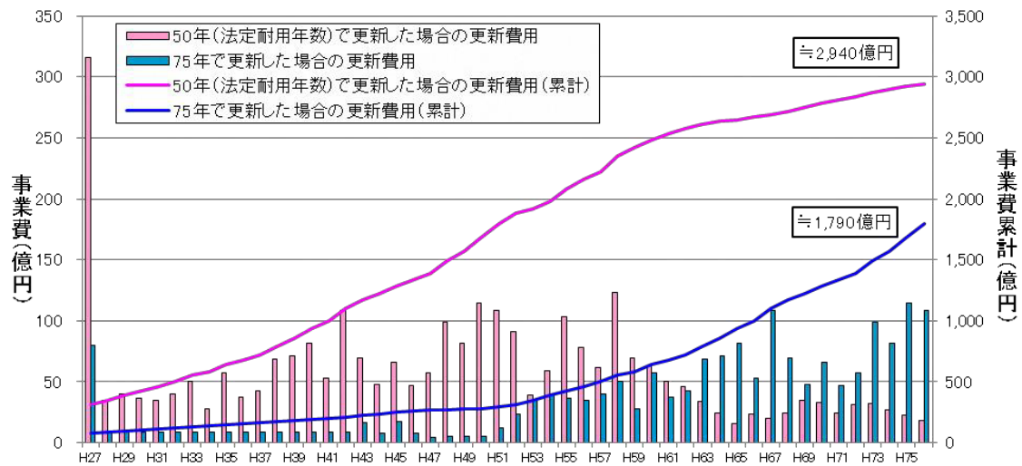
図 下水道管きよの年度別事業費の比較
