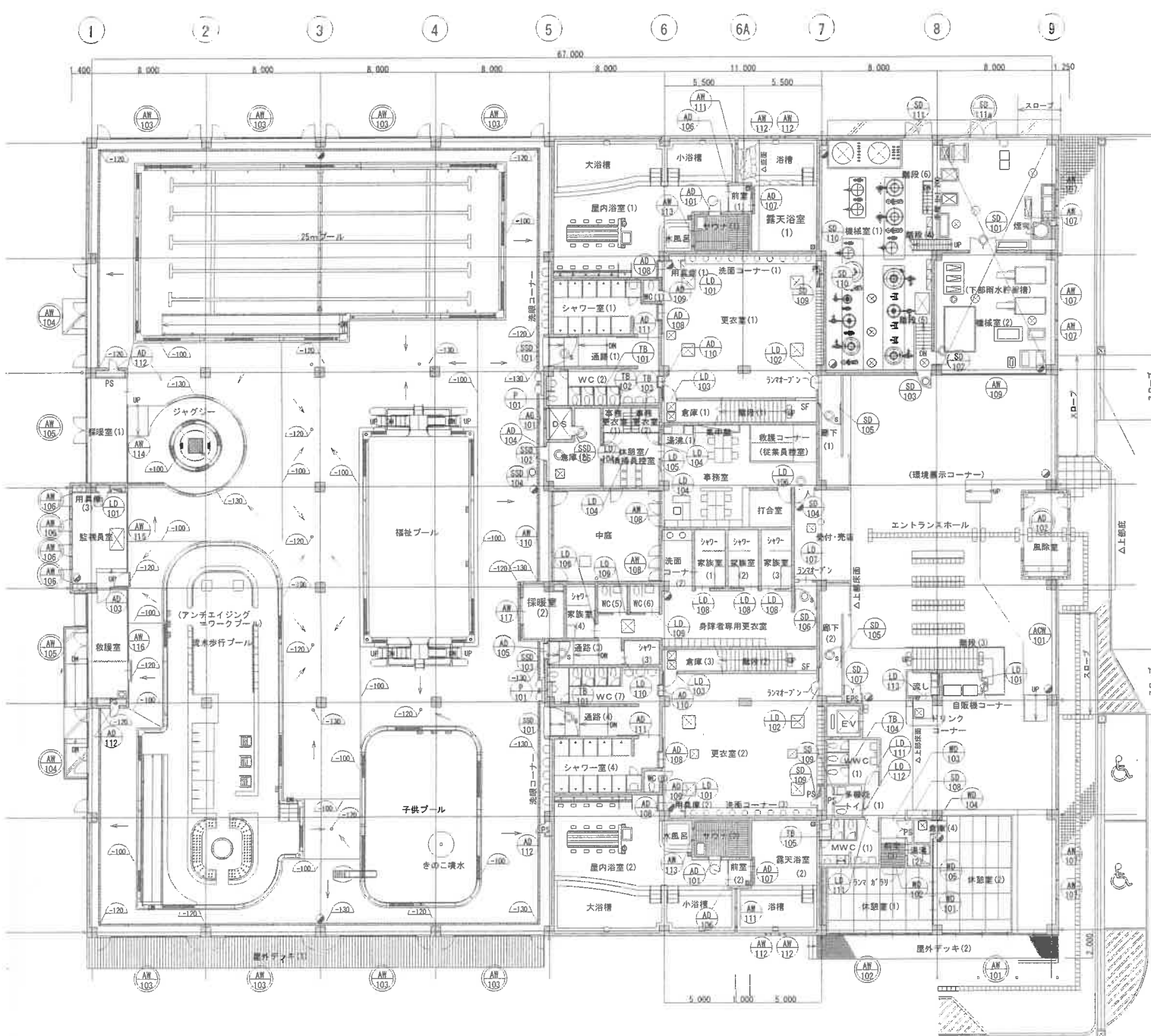
1階平面図
